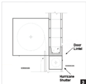
Volet anti-ouragan sous le support de linteau
