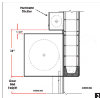
Volet anti-ouragan au-dessus du support de linteau
