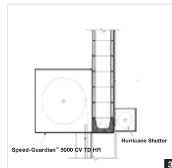
Support extérieur pour obturateur anti-ouragan
