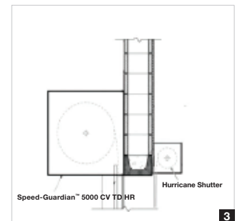
Montaje exterior de contraventana contra huracanes
