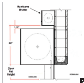
Contraventana para huracanes sobre el soporte del dintel
